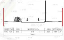
Типовой поперечный профиль улицы районного значения (ул. Лесная)
