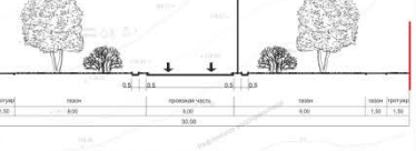
Типовой поперечный профиль магистральной улицы районного значения (ул. Парковая)
